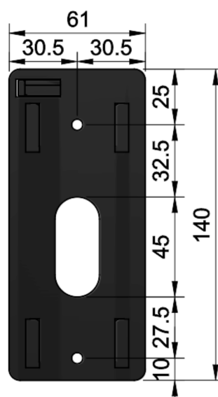
Wandhalterung
