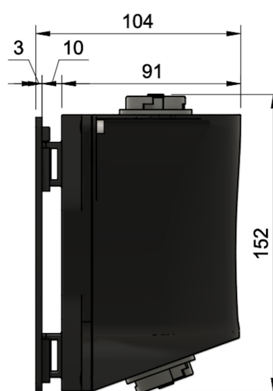
Wandhalterung
