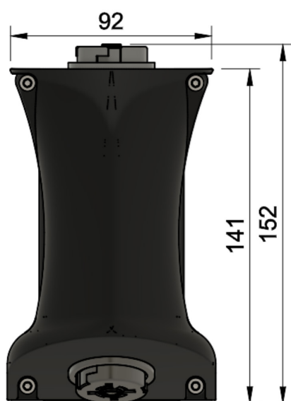
Masthalterung
