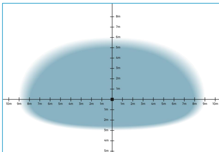
Lichtpunkthöhe: 5 Meter
